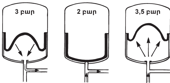
Նկար 5 Թաղանթային ճնշումային բար
