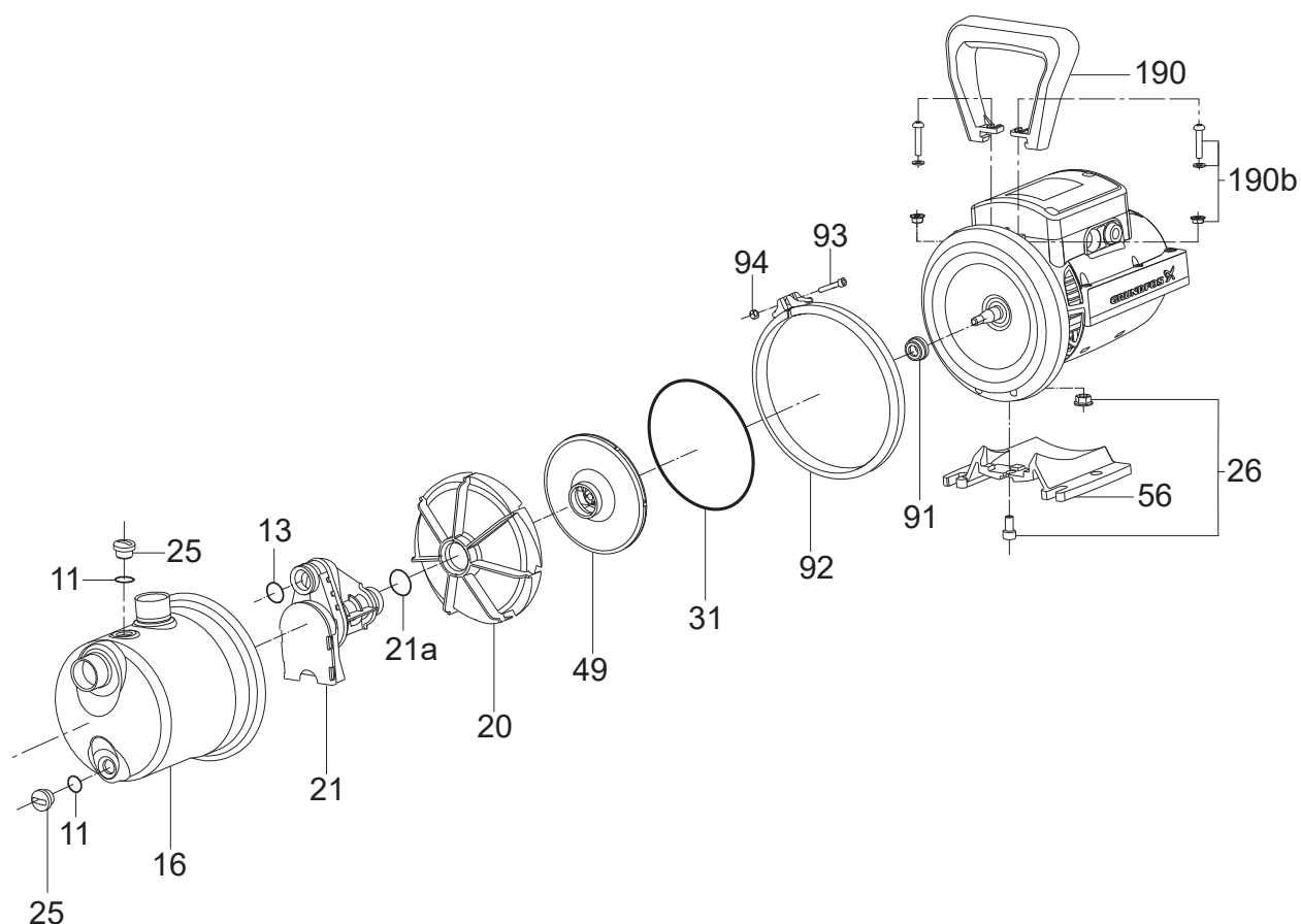
Рис. 15 Конструкция насоса JP
