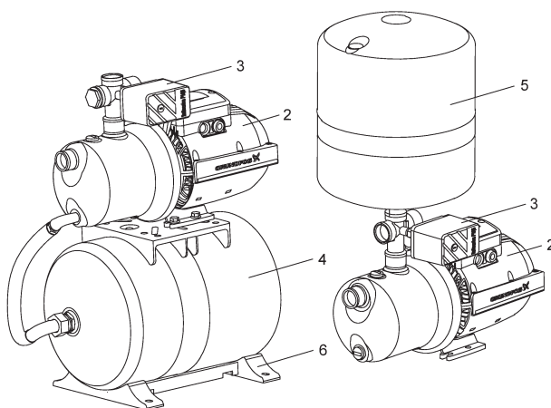
Նկար 4 JP PT-H (ծախից), JP PT-V (աջից)
