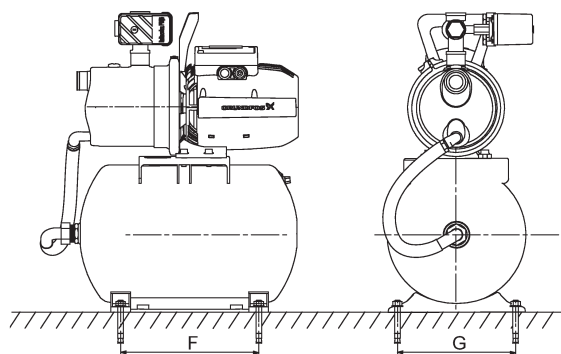
Рис. 8 Фундамент установки JP PT-H
