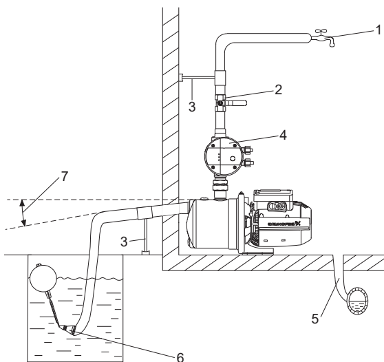
Рис. 12 Всасывание из бака/резервуара
