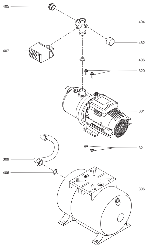
Рис. 2 Конструкция установки JP PT-H
