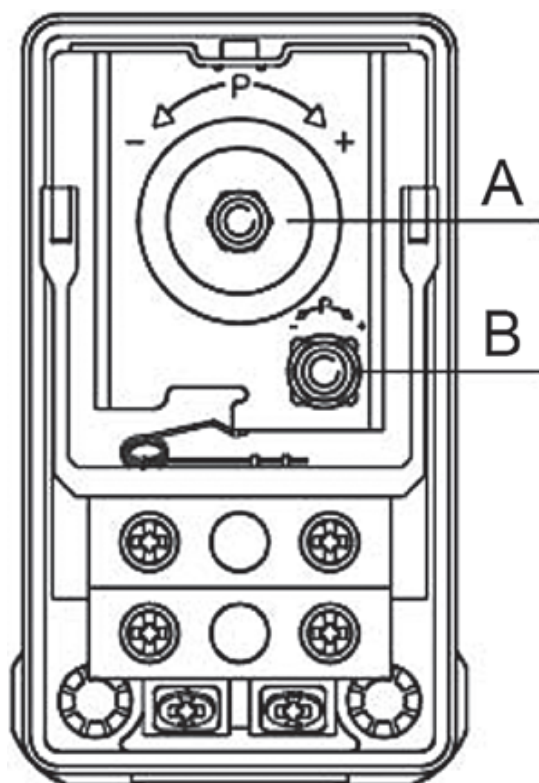
14-сур. Қысым релесі
