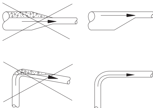
Рис. 9 Рекомендуемый монтаж трубопровода, чтобы избежать трения и скопления воздуха
