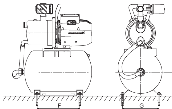
8-сүр. JP PT-H орнотуусунун пайдубалы
