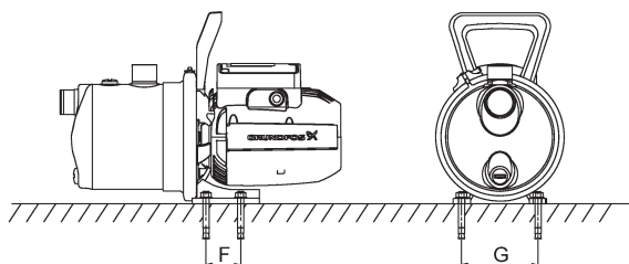
7-сур. JP сорғысының іргетасы
