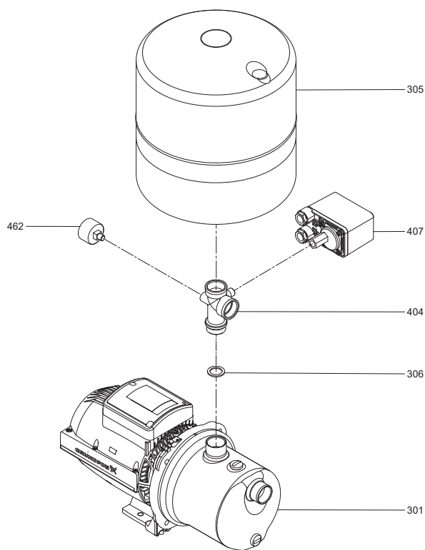
1-сүр. JP PT-V орнотуусунун түзүлүшү
