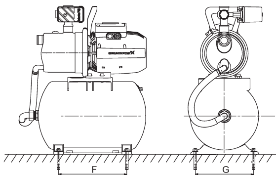
8-сур. JP PT-H қондырғысының іргетасы
