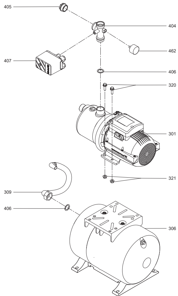
Նկար 2 JP PT-H կայանքի կառուցվածքը
