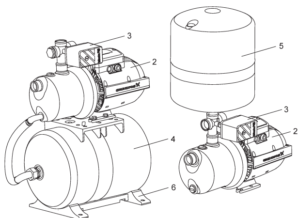
4-сур. JP RT-H (сол жақ), JP RT-H (оң жақ)
