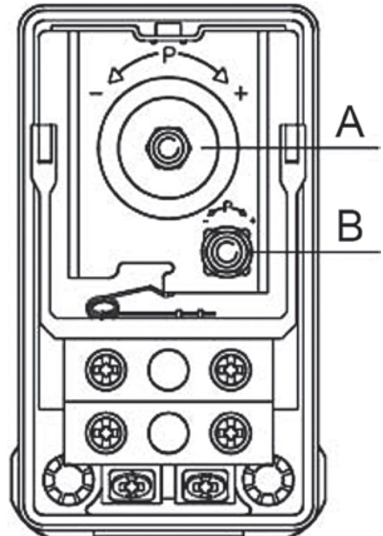
Նկար 14 Ճնշման ռելե
