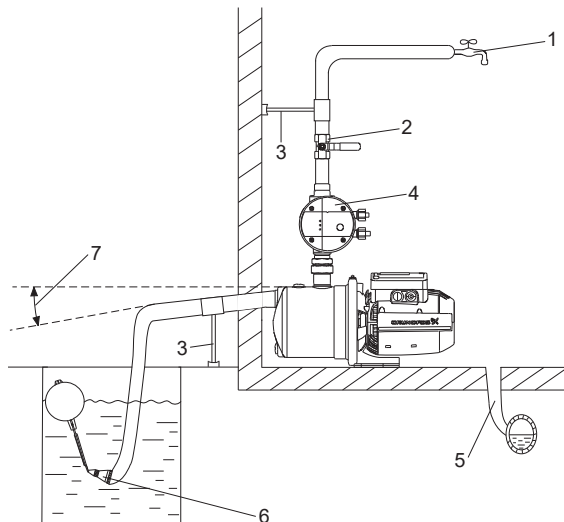
Նկար 12 Բաքից/ռեզերվուարից ներմղումը
