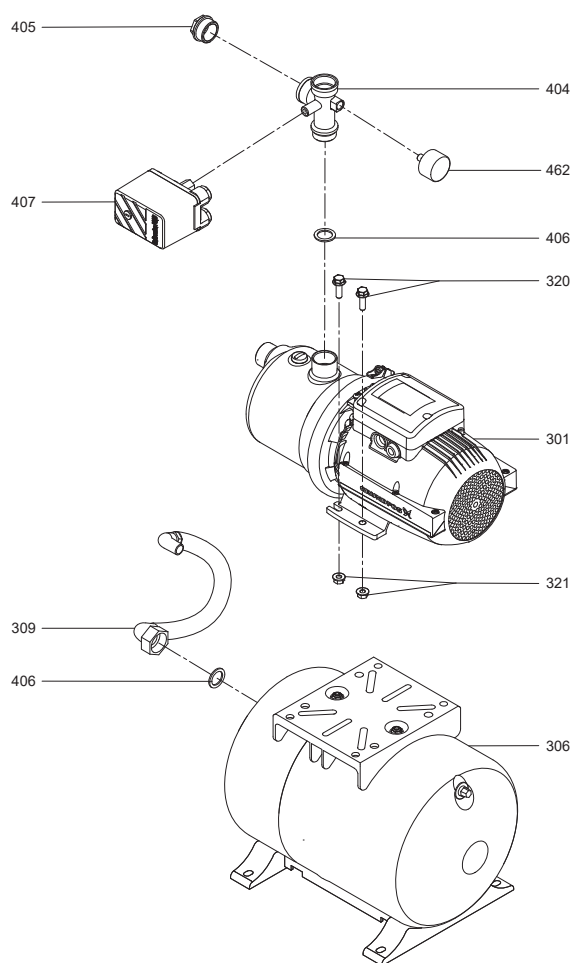
2-сүр. JP PT-H орнотуусунун түзүлүшү
