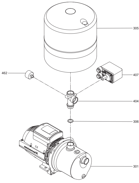
Նկար 1 JP PT-V կայանքի կառուցվածքը
