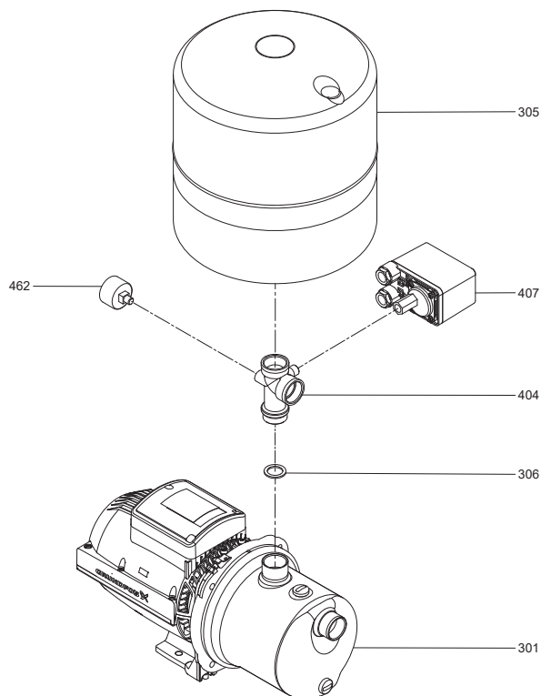
1-сур. JP PT-V қондырғысының құрылымы
