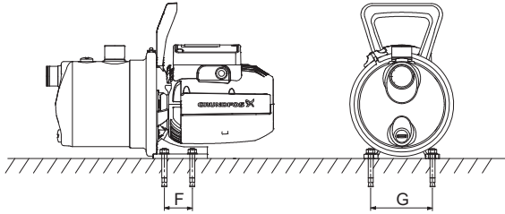
Նկար 7 JP պոմպի հիմքը
