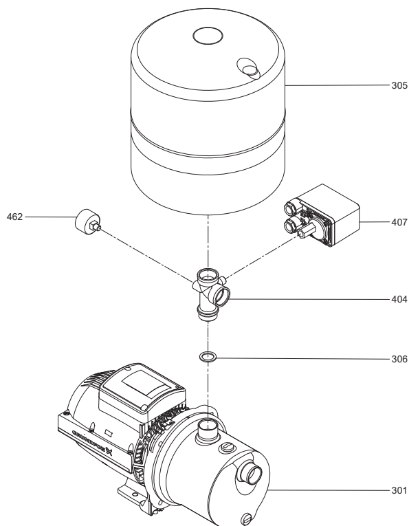
Рис. 1 Конструкция установки JP PT-V
