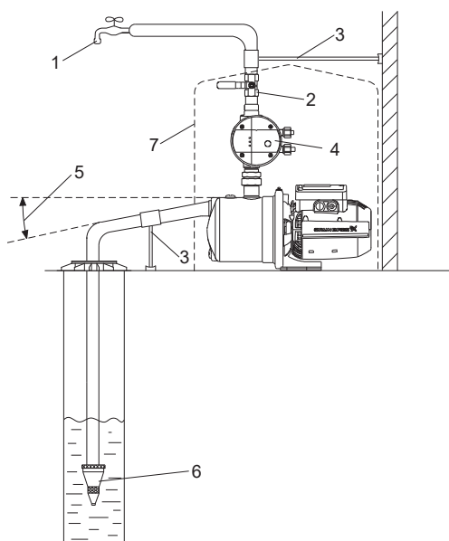
13-сүр. Сууну скважинадан чогултуу
