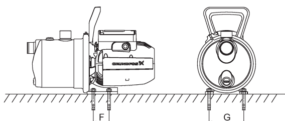
Рис. 7 Фундамент насоса JP
