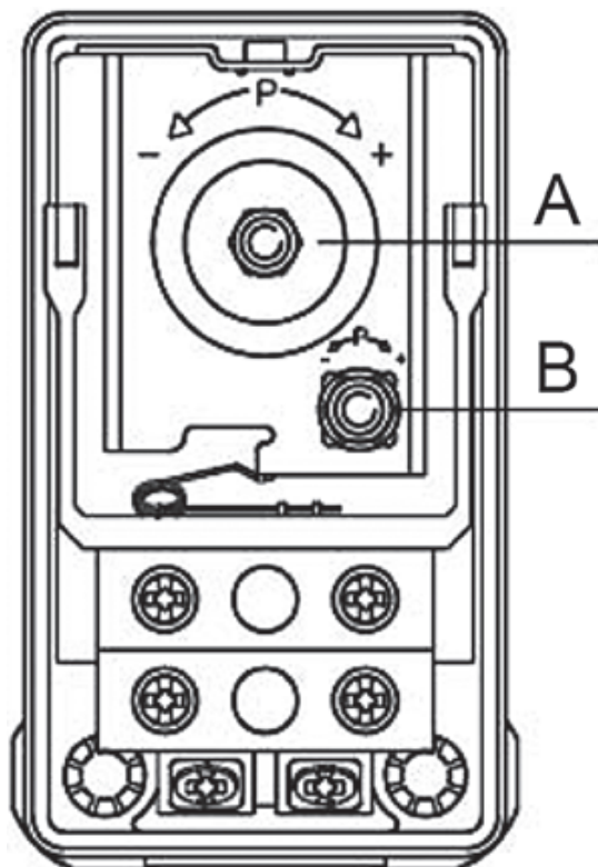
14-сүр. Басым релеси
