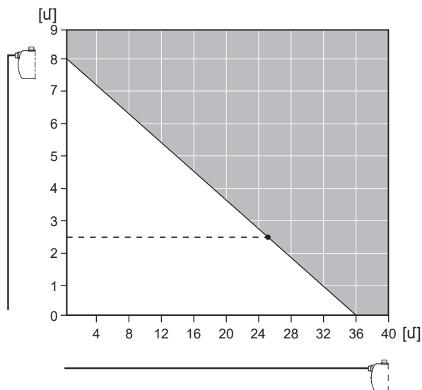
Նկար 11 Ներմղման խողովակաշարի առավելագույն երկարությունը (հորիզոնական առանցք) կախված ներմղման բարձրությունից (ուղղաձիգ առանցք)
