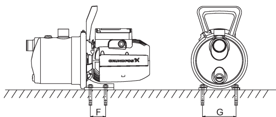
7-сүр. JP соркысмасынын фундаменти
