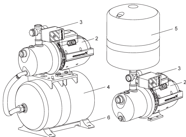
Рис. 4 JP PT-H (слева), JP PT-V (справа)
