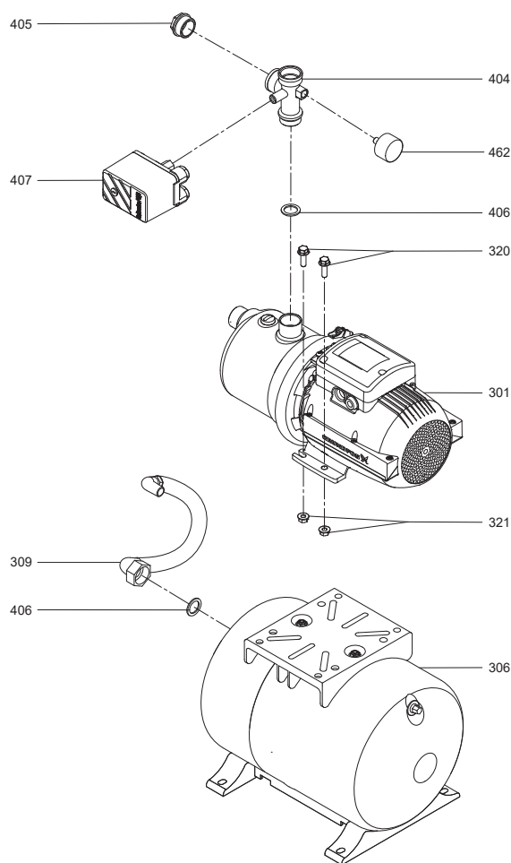
2-сур. JP PT-H қондырғысының құрылымы
