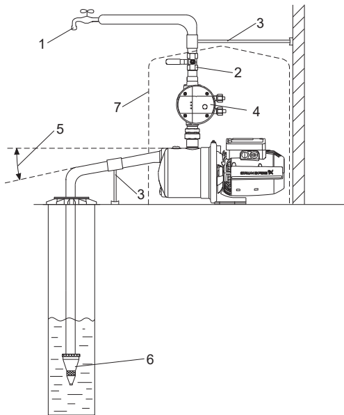
Նկար 13 Հորատանցքից ջրի մատակարարում
